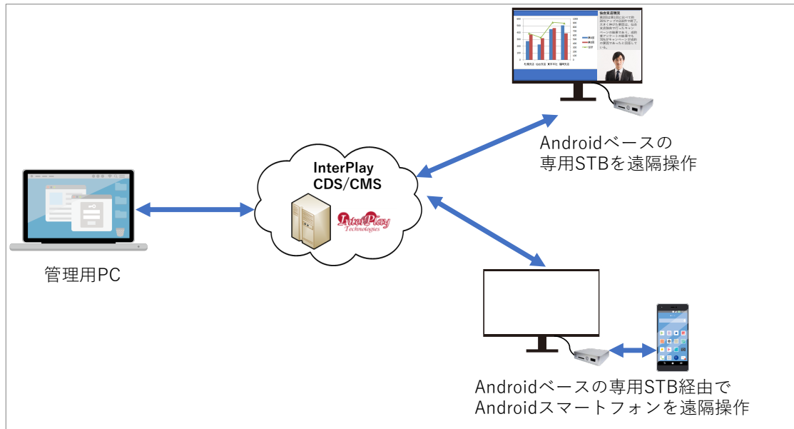
■InterPlayMDM システム構成図
